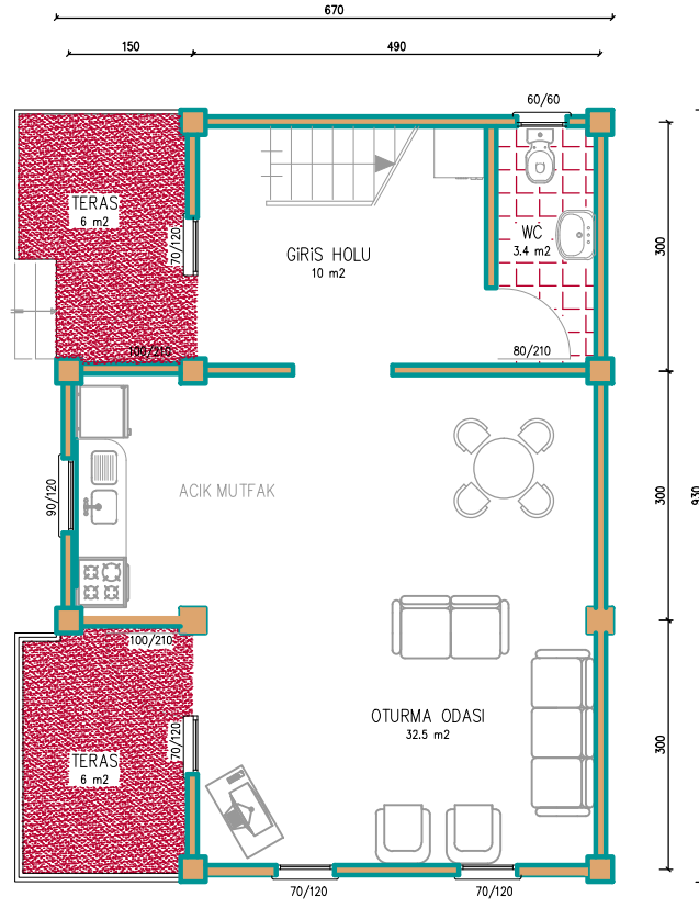
ZEMİN KAT PLANI
